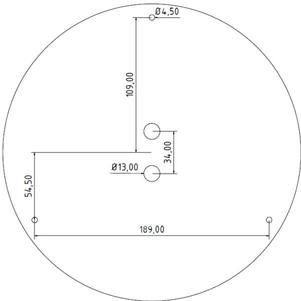
Montagemaße 58271000
