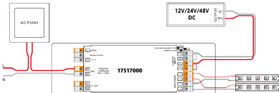
Abb. 03 - Anschluss Push-Dimm
