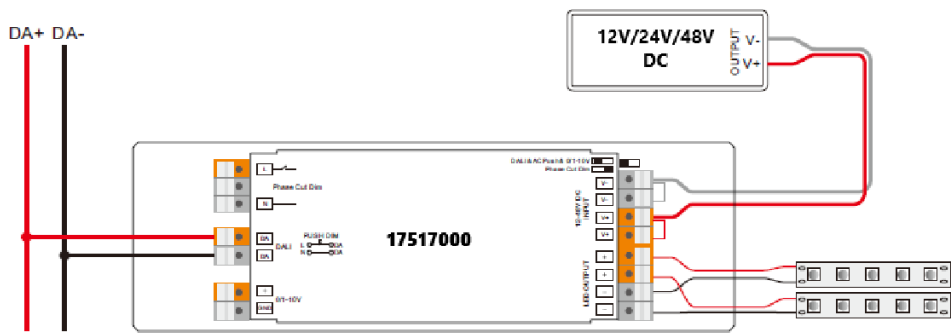
Abb. 02 - Anschluss DALI-Bus
