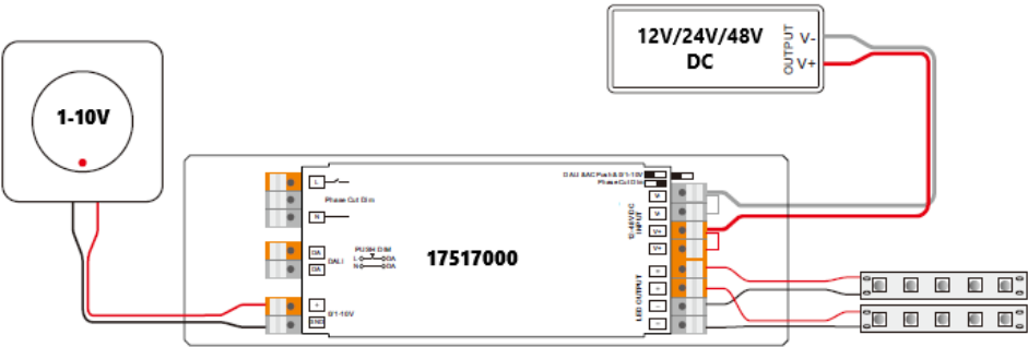
Abb. 04 - Anschluss 1-10V
