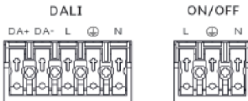
Anschlussschema: Dali oder schaltbar
