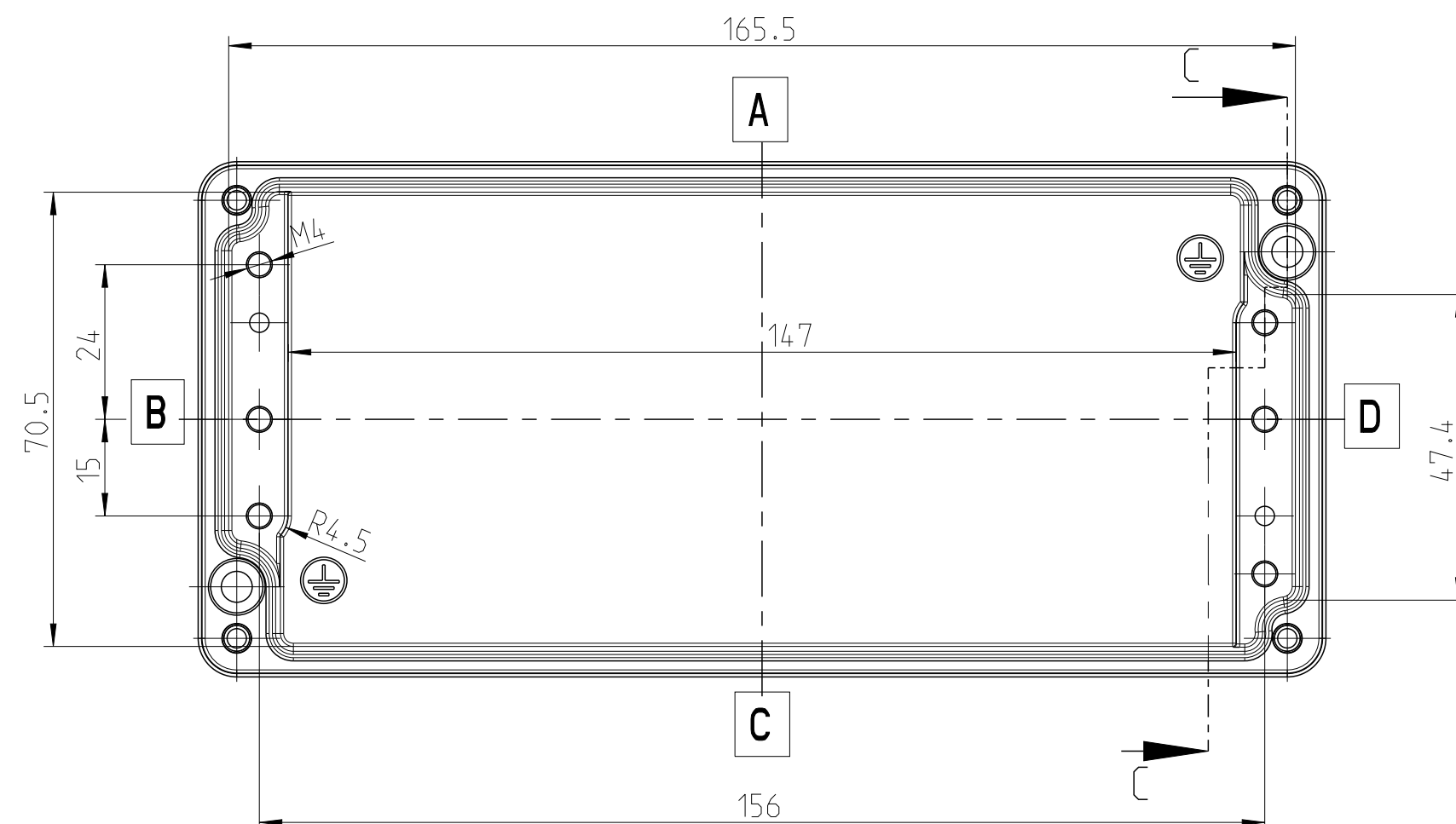
Innenansicht Unterteil/ interior view bottom part
