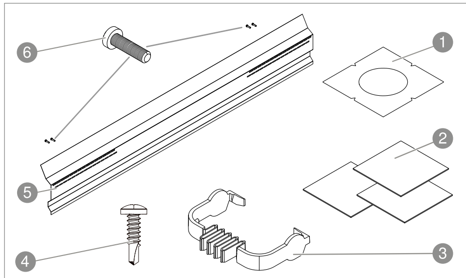
Abb. 4: Systemzubehör
