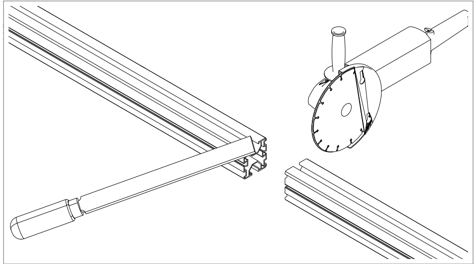
Abb. 7: Trägerprofil ablängen
