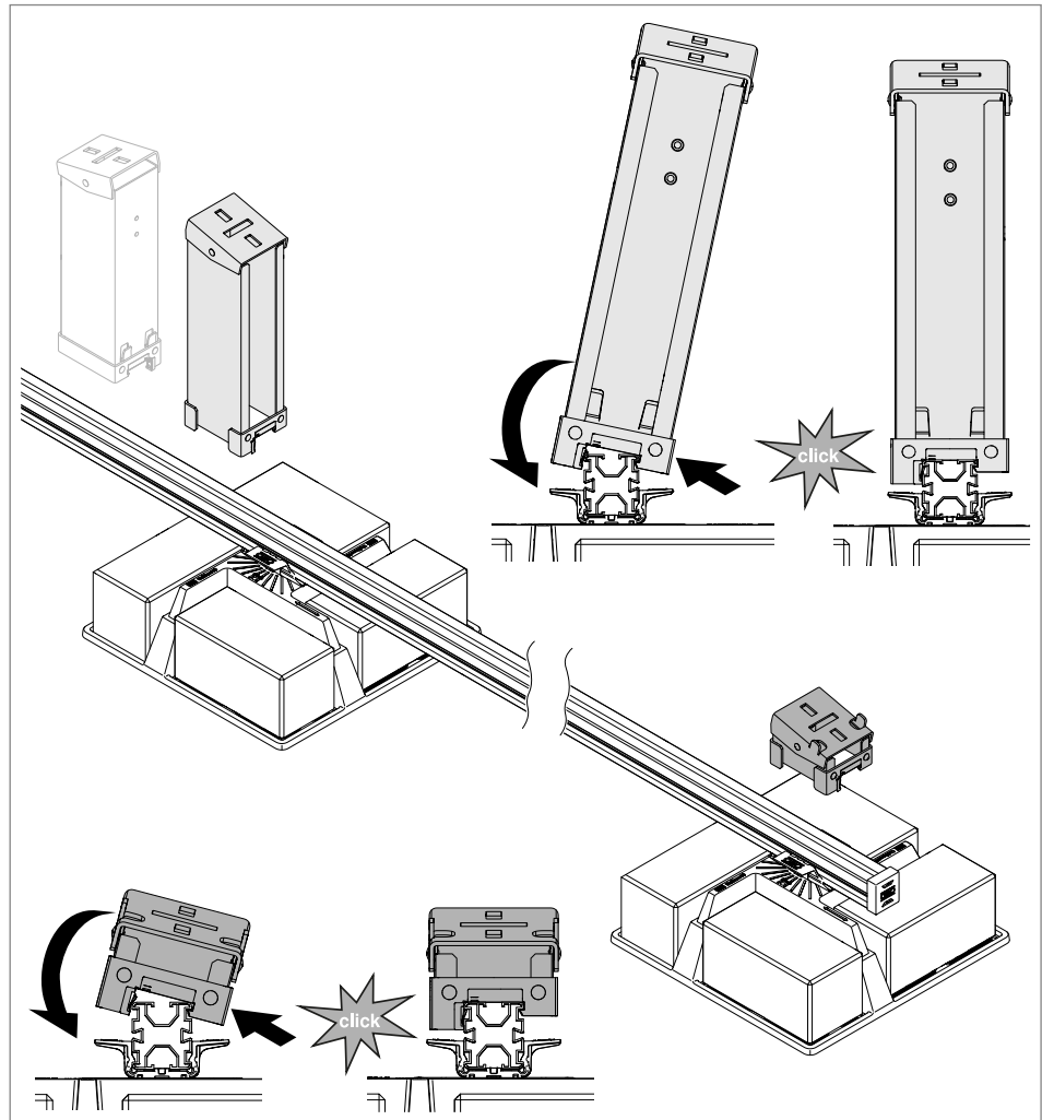
Abb. 12: Stützen einsetzen
