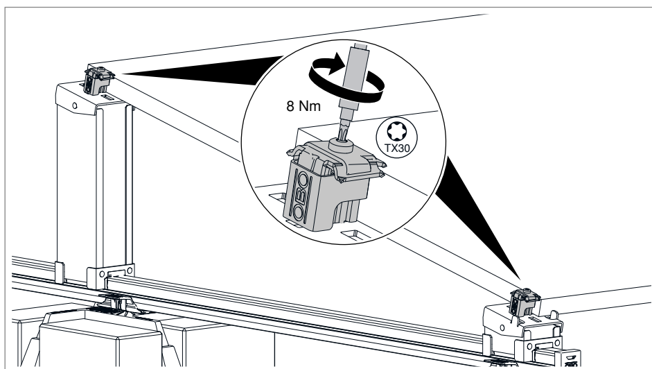
Abb. 18: Universalklemmen befestigen
