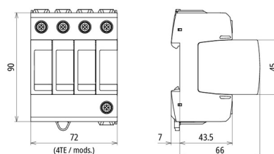
Maßbild DG MD TNS 275
