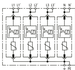
Prinzipschaltbild DG MD TNS 275
