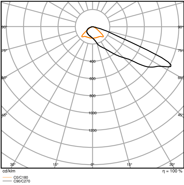
FL MAX P 600W 857 A65x120 WAL
