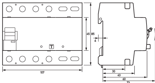
Maßzeichnung Gruppenansicht
