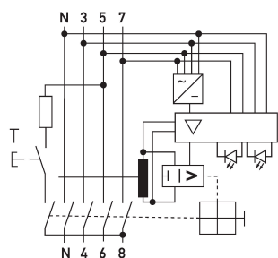
Anschlusschema
