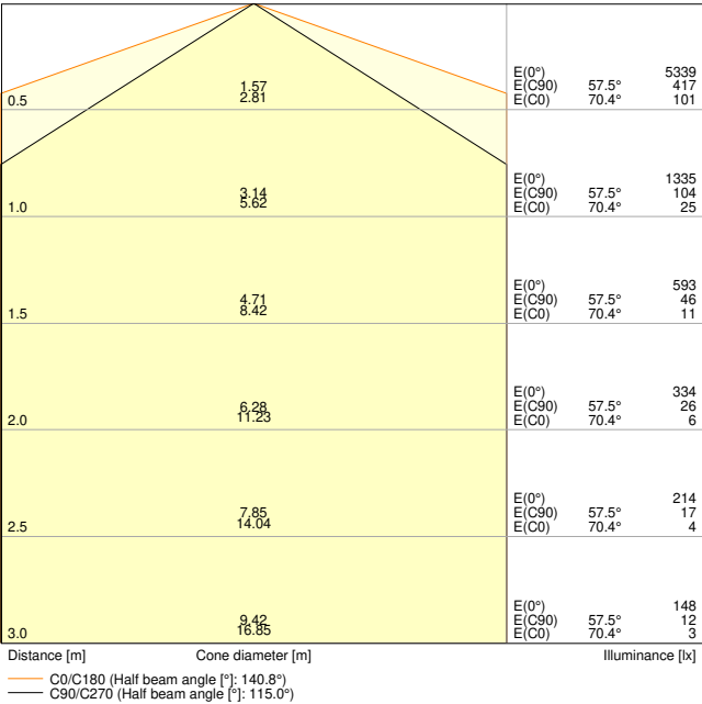
DP SLIM 1500 V 39W ML 865 IP65
