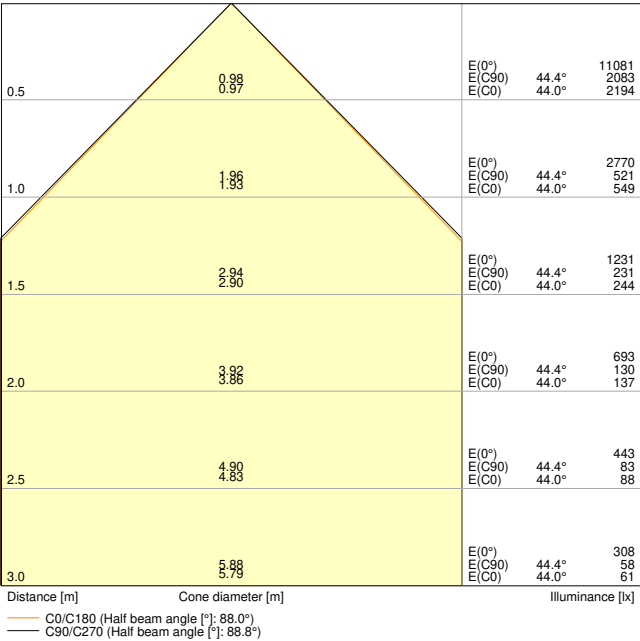
PL INV 600 DA P 38W ML 940 U19 WT
