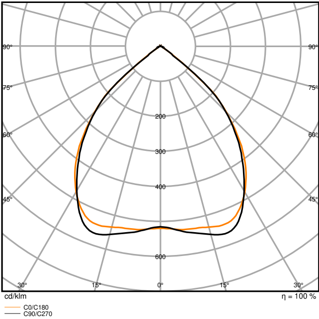
PL INV 600 ZB P 38W 930 U19 WT-800mA
