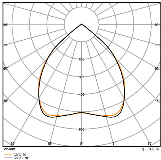
PL INV 1200 ZB P 38W 930 U19 BK-800mA
