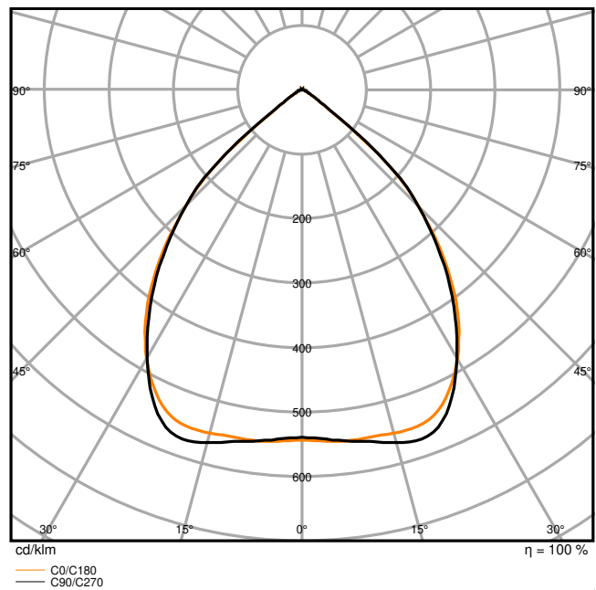
PL INV 1200 ZB P 38W 940 U19 WT-800mA
