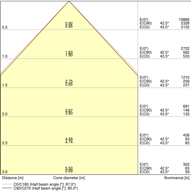
PL INV 1200 ZB P 38W 940 U19 BK-800mA
