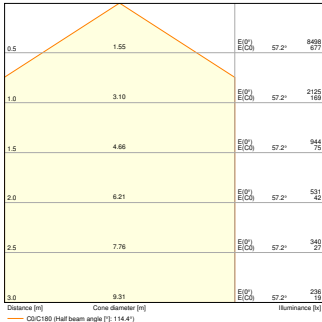
PL SF 1574 DA V 48W 940 6240lm
