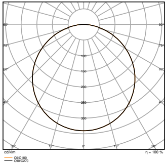
PL SF 1574 DA V 48W 930 6240lm
