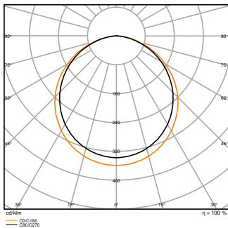
PL COMP 1200 DA V 30W 830 4200lm
