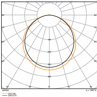
PL COMP 1200 DA V 30W 840 4200lm
