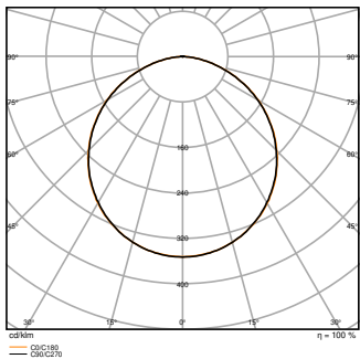
PL COMP 600 DA V 30W 840 4200lm
