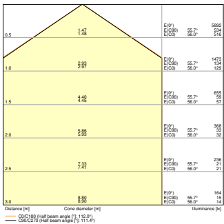
PL COMP 600 DA V 30W 865 4200lm
