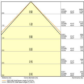
PL COMP 625 DA V 30W 865 U19 4200lm
