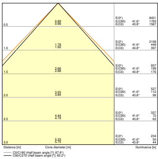
PL COMP 625 DA V 30W 840 U19 4200lm
