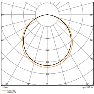
PL COMP 1200X600 DA V 44W 830 5880lm
