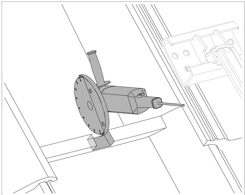
Abb. 12: Ziegel aussparen
