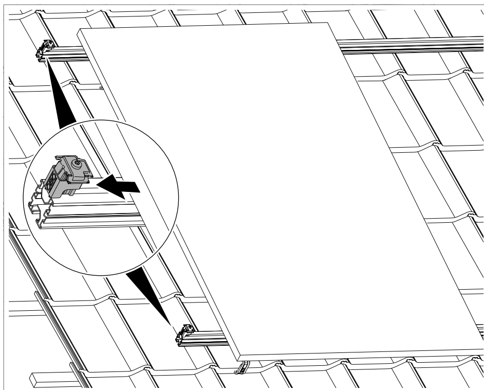
Abb. 30: PV-Modul auflegen
