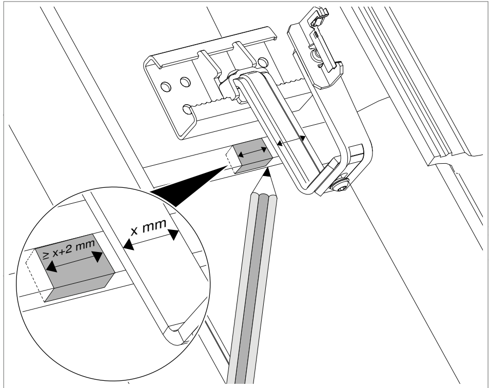
Abb. 11: Aussparung anzeichnen
