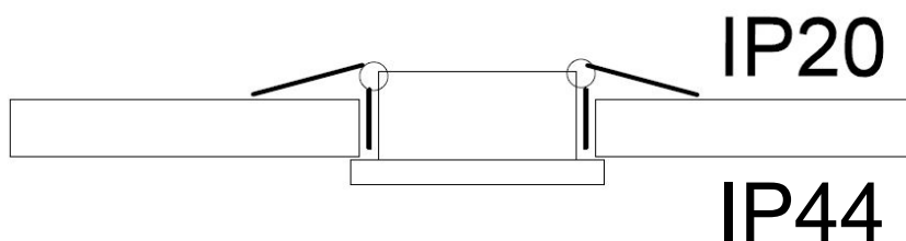
Abb.: 2 Einbau in geschlossene Decken
