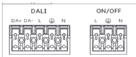
Abb.: 3 Anschlussschema: Dali oder schaltbar
