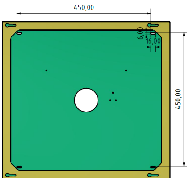
Abb.: 1 Montageplatte Lochmaße
