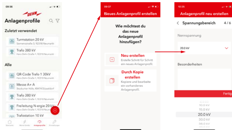
Bild 10 Anlagenprofil neu erstellen
