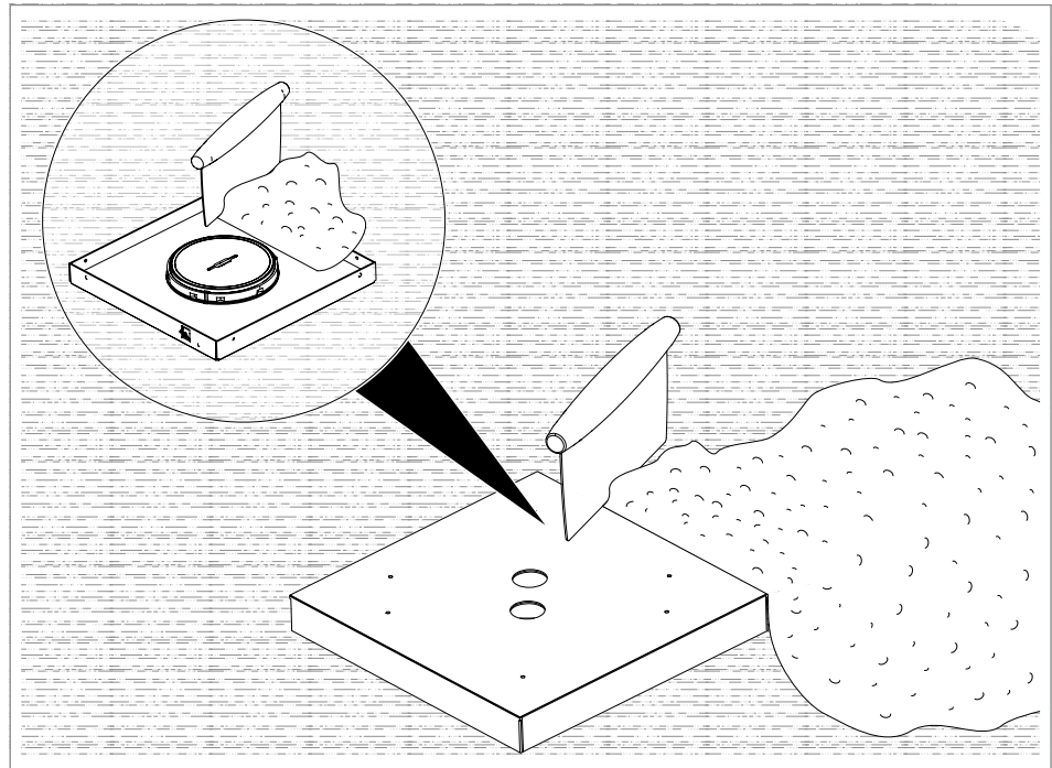
Abb. 17: Terrazzobelag aufbringen
