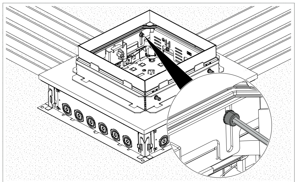
Abb. 11: Feinnivellierung Kassette
