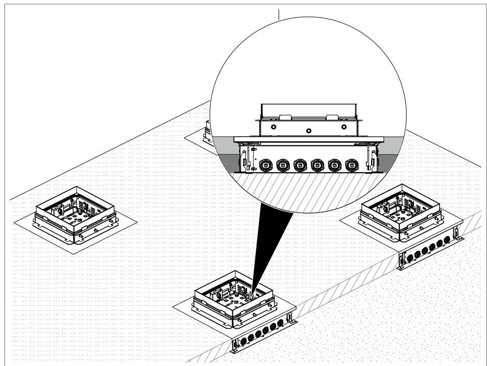
Abb. 12: Dämmung/Trittschall einbringen
