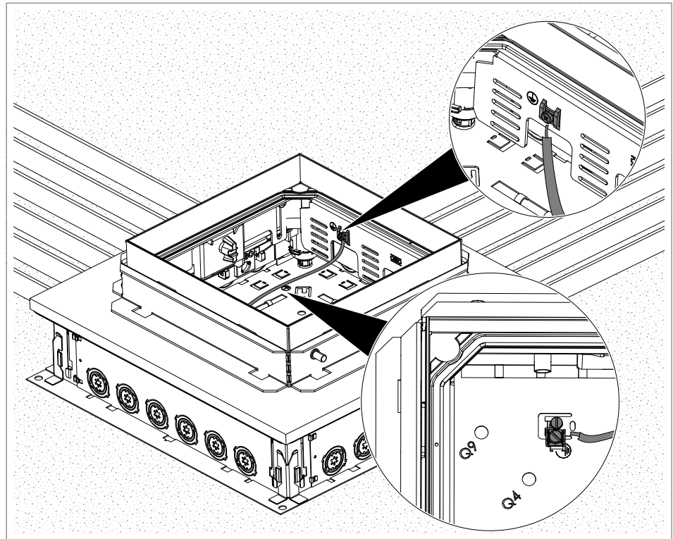
Abb. 10: Potentialausgleich herstellen
