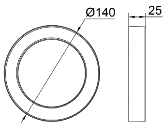
Artikel-Nr. 5620-40-0003 6 W LED, 450 lm Ø 140 x 25 mm, 0,22 kg für Lochausschnitt: Ø von 55 mm bis 110 mm □ von 55x30 mm bis 80x80 mm
