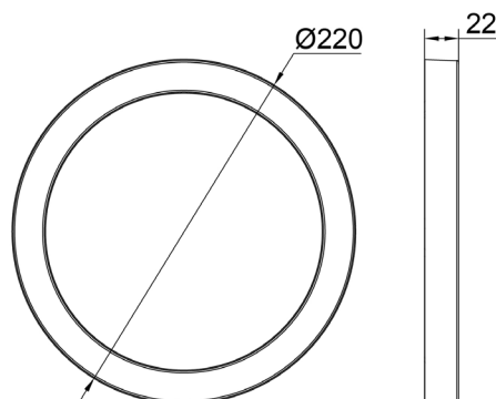
Artikel-Nr. 5620-40-0005 18 W LED, 1440 lm Ø 220 x 22 mm, 0,45 kg für Lochausschnitt: Ø von 55 mm bis 200 mm □ von 55x30 mm bis 130x130 mm
