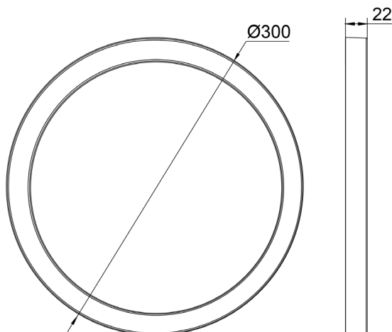
Artikel-Nr. 5620-40-0006 24 W LED, 1920 lm Ø 300 x 22 mm, 0,60 kg für Lochausschnitt: Ø von 55 mm bis 270 mm □ von 55x30 mm bis 180x180 mm
