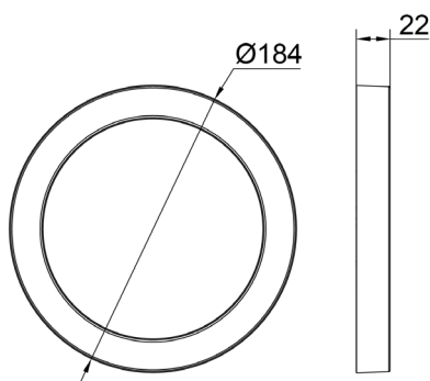
Artikel-Nr. 5620-40-0004 12 W LED, 960 lm Ø 184 x 22 mm, 0,30 kg für Lochausschnitt: Ø von 55 mm bis 160 mm □ von 55x30 mm bis 110x110 mm
