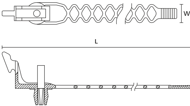
Befestigungsbinder FBR
