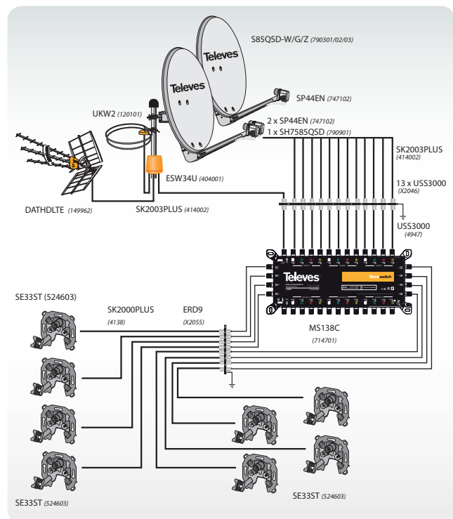
Anlage für 8 Teilnehmer: 3 Satelliten Astra 19°, Hotbird 13° und Eutelsat 9° + DVB-T + UKW
