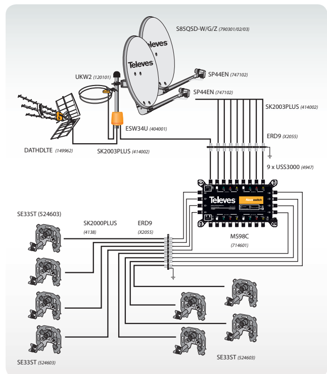
Anlage für 8 Teilnehmer: 2 Satelliten Astra 19° und Hotbird 13° + DVB-T + UKW
