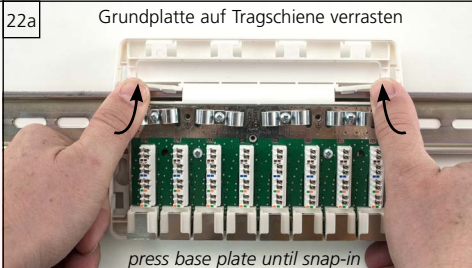
Grundplatte mit Tragschienen-Adapter auf Tragschiene verrasten
