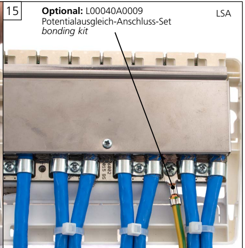
Optional: L00040A0009 Potentialausgleich-Anschluss-Set bonding kit
