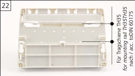
Optional: DIN Tragschienen-Adapter / DIN mounting rail adapter 2xH06000A0056
