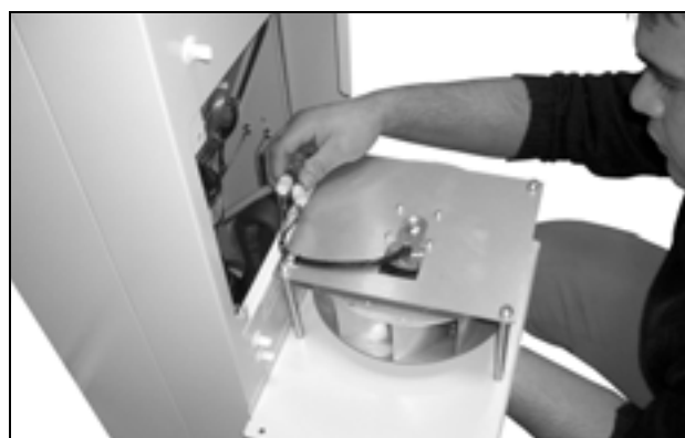
Fig. 70: Desencaixar os conectores do ventilador (1)
