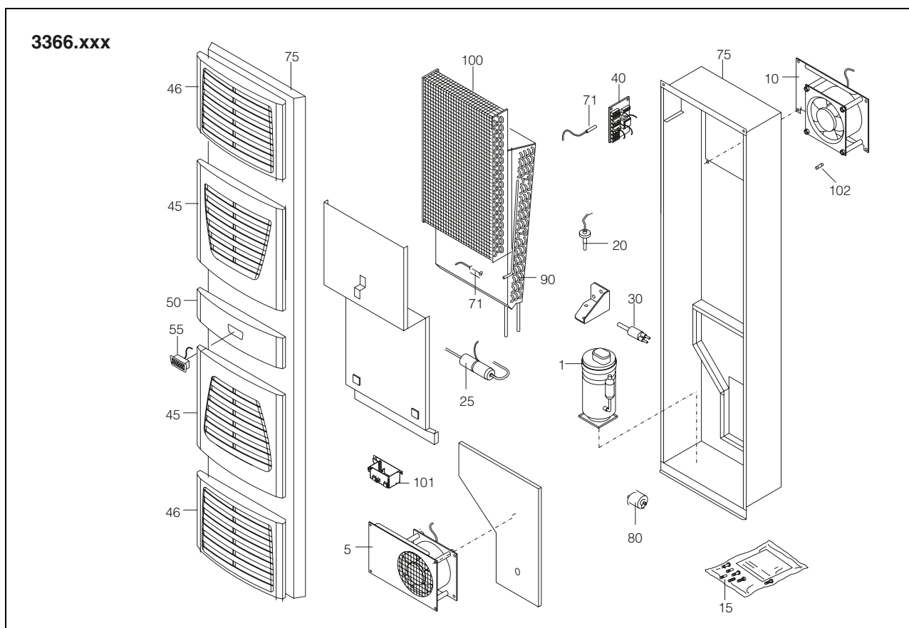
Fig. 123: Peças de reposição para os modelos 3366.xxx
