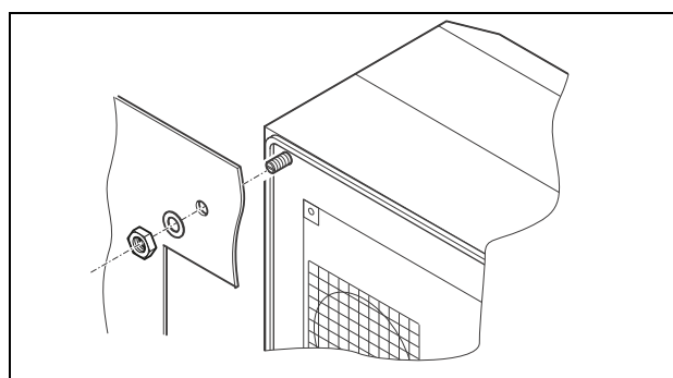
Fig. 9: Fixar o aparelho (apenas 3302.1xx "montagem externa")
