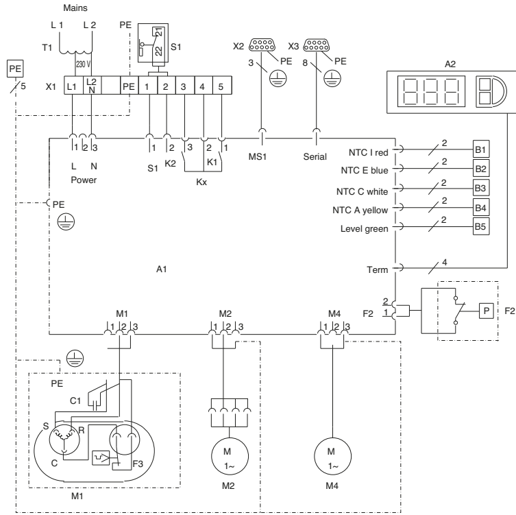
Fig. 25: Esquema de conexões elétricas nº 3
