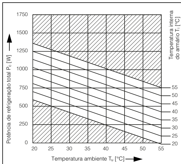
Fig. 92: 3303.xxx, 500 W, 60 Hz
