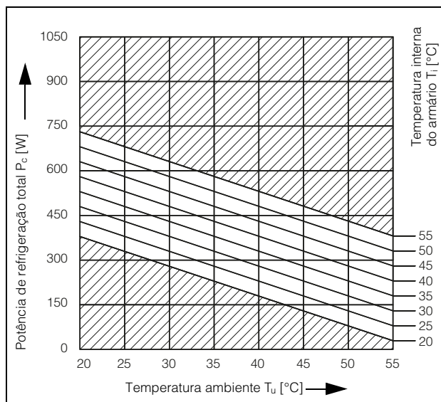
Fig. 90: 3302.xxx, 300 W, 60 Hz
