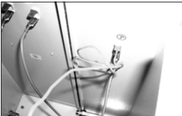
Fig. 73: Desencaixar o cabo de aterramento do ventilador (1)
