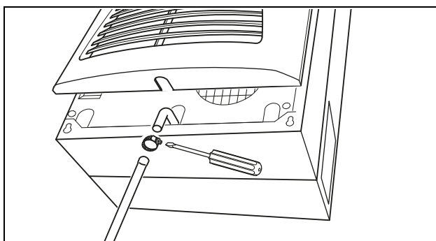
Fig. 19: Conexão da saída para a água condensada
