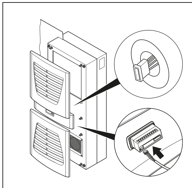
Fig. 14: Encaixar o conector do display
