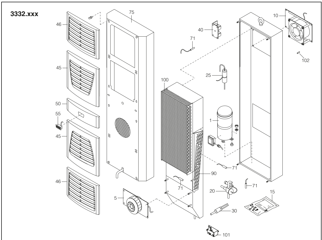
Fig. 122: Peças de reposição para os modelos 3332.xxx
