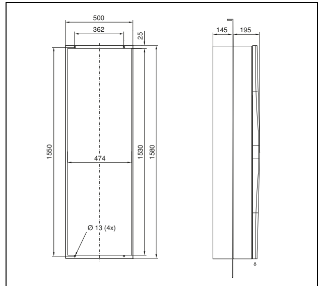
Fig. 137: 3332.xxx para montagem interna parcial
