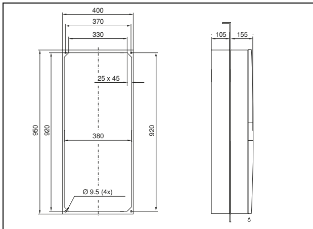
Fig. 135: 3304.xxx, 3305.xxx para montagem interna parcial
