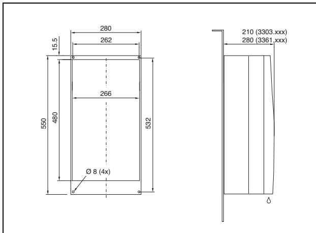
Fig. 126: 3303.xxx, 3361.xxx para montagem externa (exceto os aparelhos NEMA 4X)
