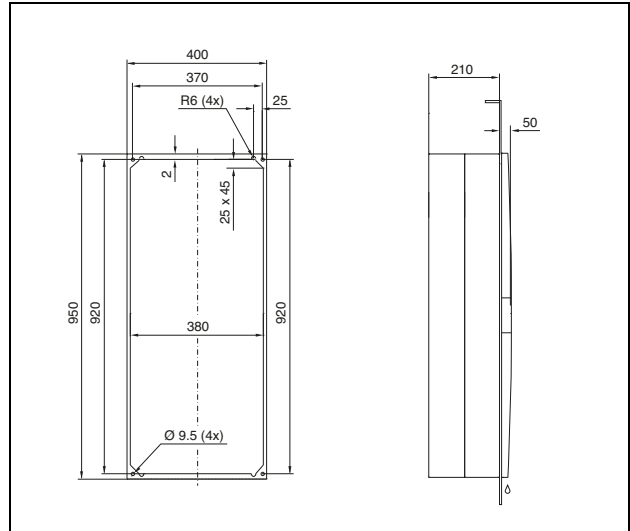
Fig. 141: 3304.xxx, 3305.xxx para montagem interna total
