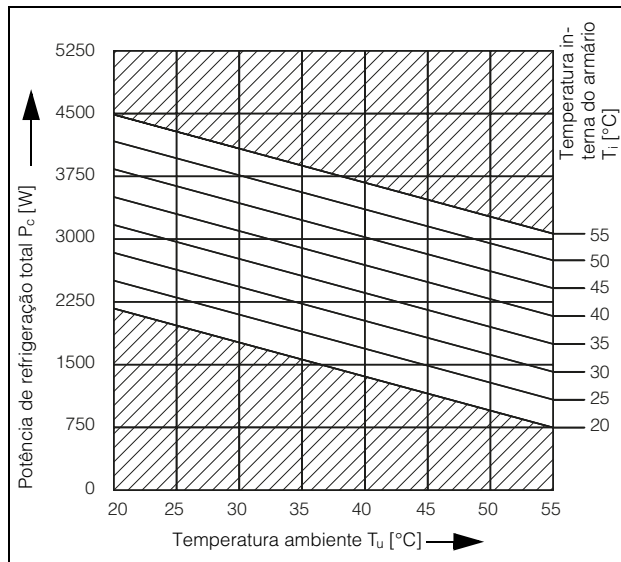
Fig. 102: 3328.xxx, 2000 W, 60 Hz
