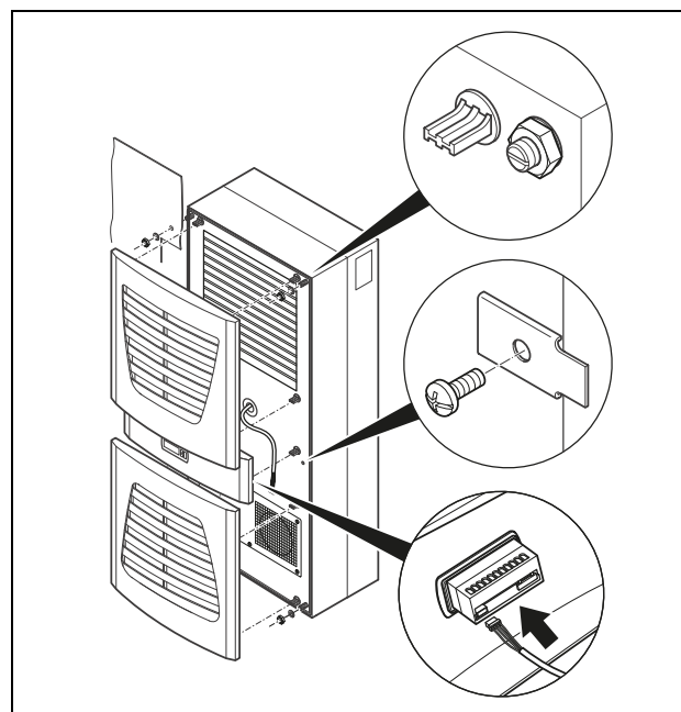
Fig. 18: Fixar o condicionador de ar
