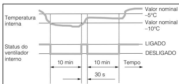
Fig. 36: Diagrama do modo ECO
