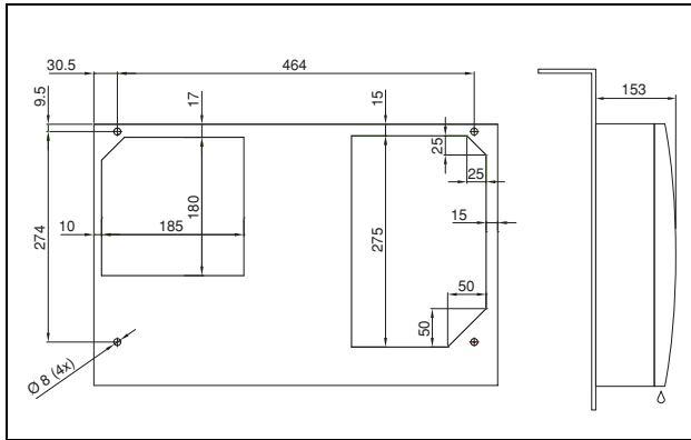
Fig. 125: 3302.3xx para montagem externa
