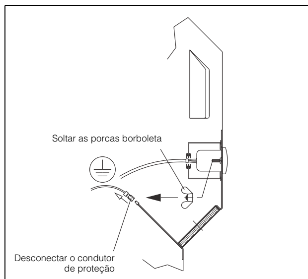
Fig. 85: Remoção da tampa (2)
