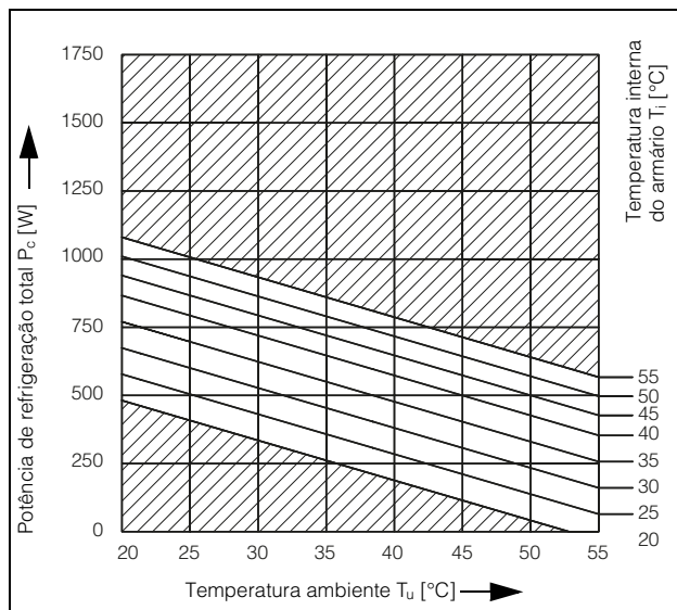
Fig. 91: 3303.xxx, 500 W, 50 Hz
