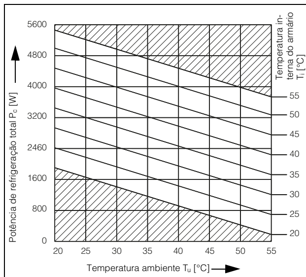
Fig. 104: 3329.xxx, 2500 W, 60 Hz
