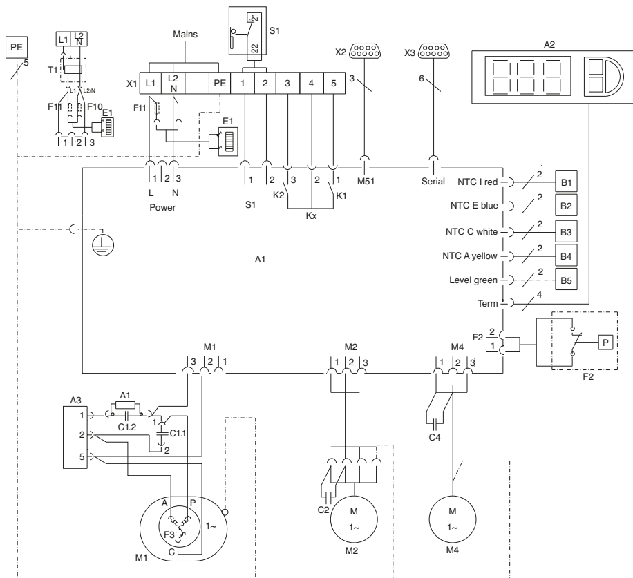
Fig. 29: Esquema de conexões elétricas nº 7
