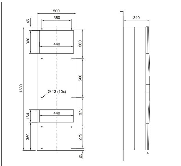
Fig. 130: 3332.xxx para montagem externa
