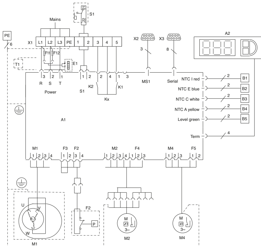
Fig. 30: Esquema de conexões elétricas nº 8
