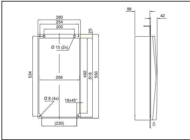
Fig. 138: 3302.xxx para montagem interna total (exceto 3302.3xx)
