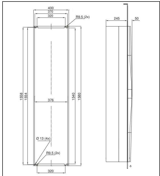
Fig. 142: 3328.xxx, 3329.xxx para montagem interna total
