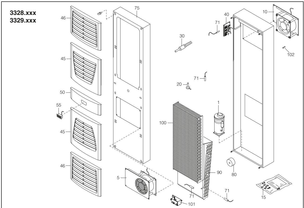
Fig. 121: Peças de reposição para os modelos 3328.xxx, 3329.xxx
