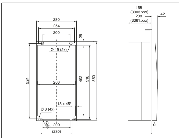
Fig. 140: 3303.xxx, 3361.xxx para montagem interna total
