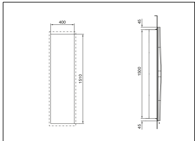
Fig. 143: 3366.xxx para montagem interna total
