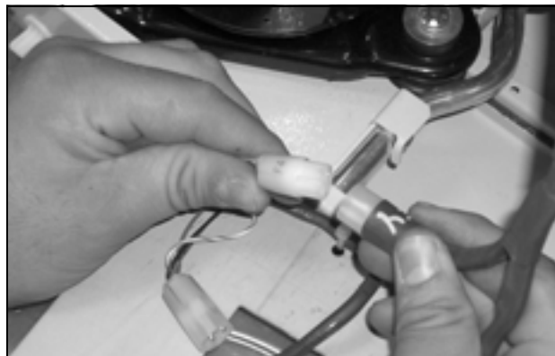
Fig. 48: Desencaixar os conectores do ventilador
