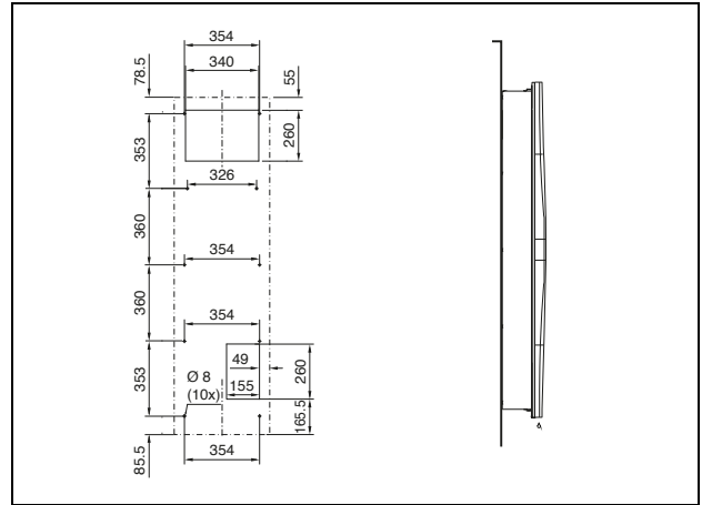
Fig. 127: 3366.xxx para montagem externa
