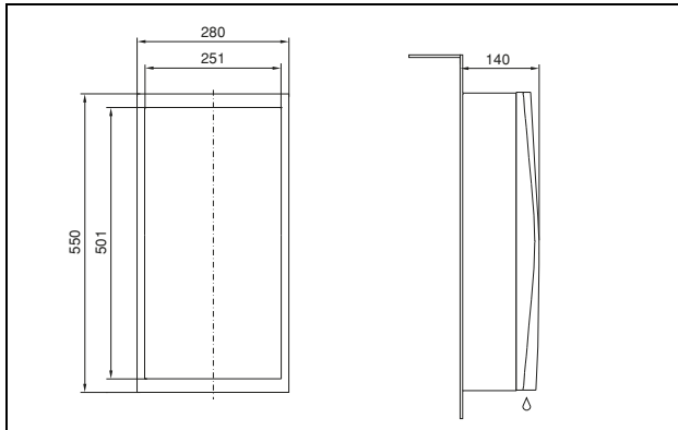
Fig. 124: 3302.xxx para montagem externa (exceto 3302.3xx)
