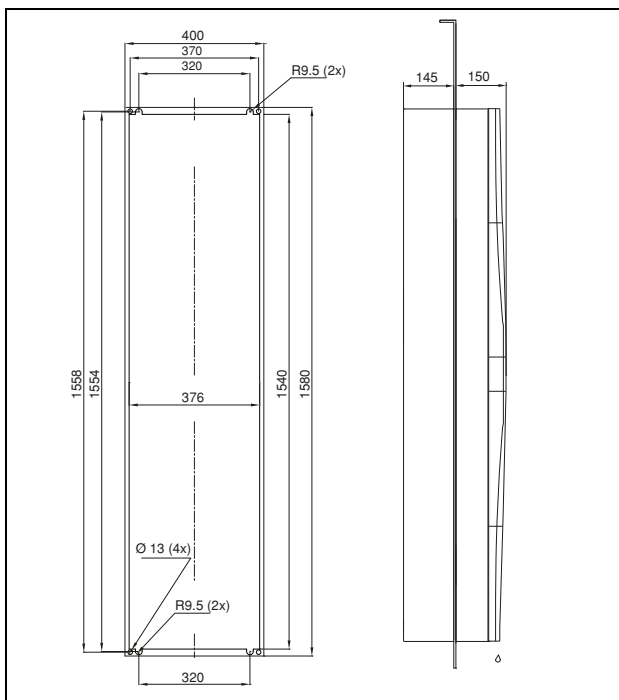
Fig. 136: 3328.xxx, 3329.xxx para montagem interna parcial
