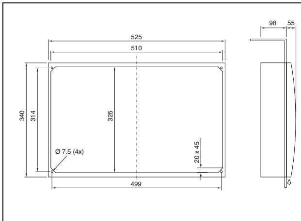
Fig. 139: 3302.3xx para montagem interna total
