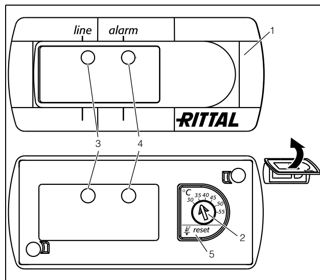
Fig. 33: Controlador básico
