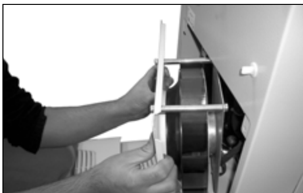
Fig. 47: Retirar o ventilador
