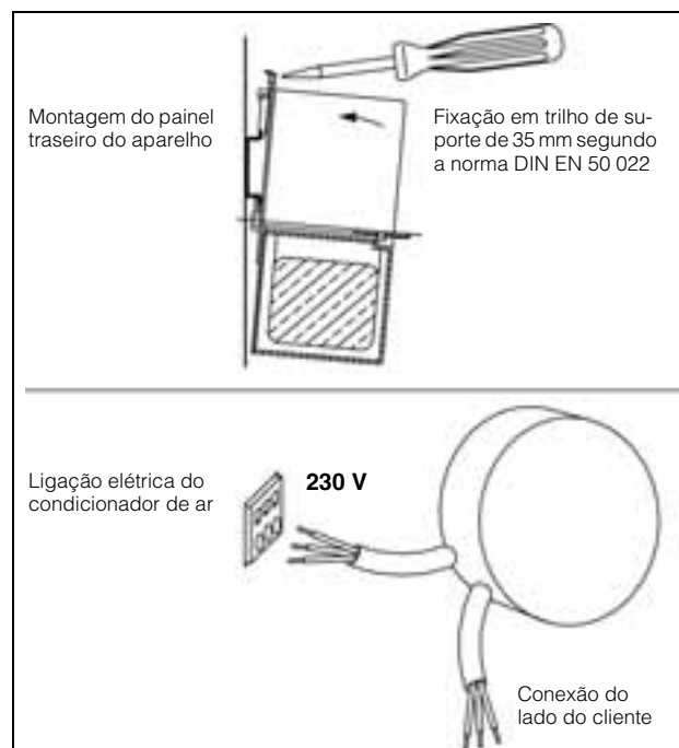
Fig. 20: Montagem de transformador externo (apenas 3361.x40)
