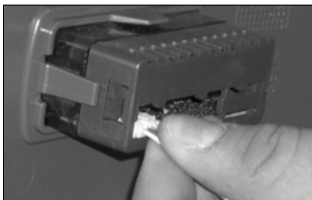
Fig. 44: Desencaixar o conector do display (2)
