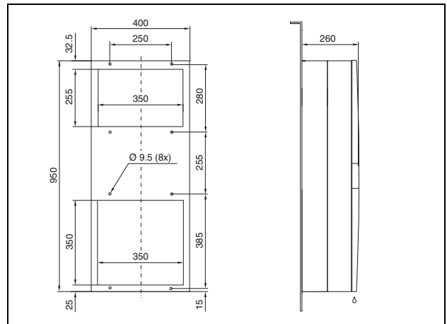
Fig. 128: 3304.xxx, 3305.xxx para montagem externa (exceto os aparelhos NEMA 4X)
