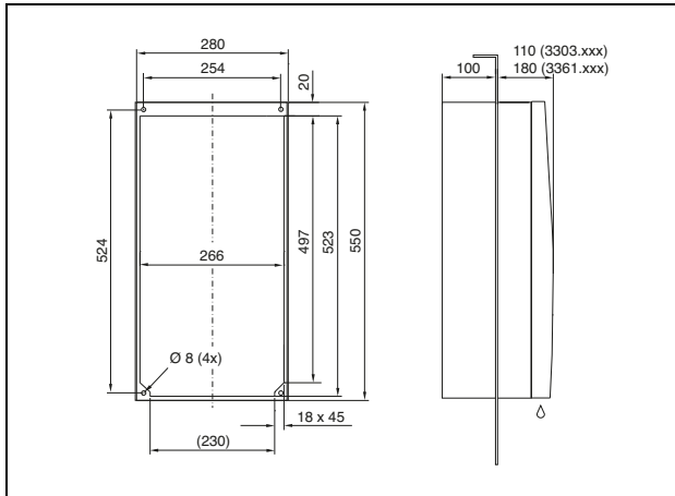
Fig. 134: 3303.xxx, 3361.xxx para montagem interna parcial
