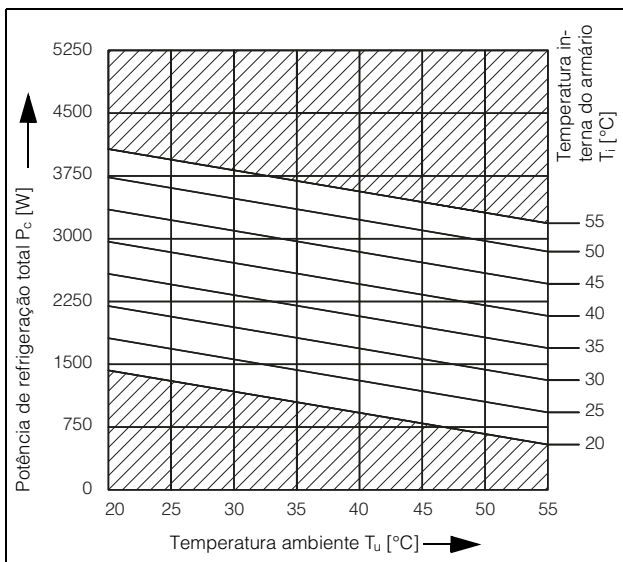
Fig. 101: 3328.xxx, 2000 W, 50 Hz
