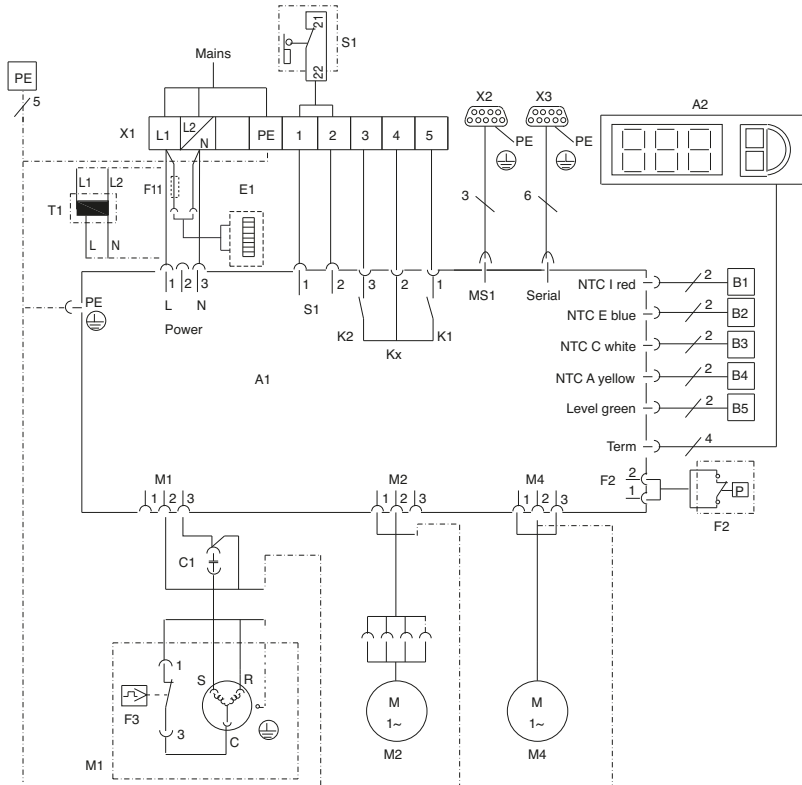
Fig. 26: Esquema de conexões elétricas nº 4
