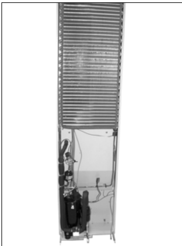
Fig. 79: Limpar os tubos do trocador de calor e o compartimento do compressor com ar comprimido (1)
