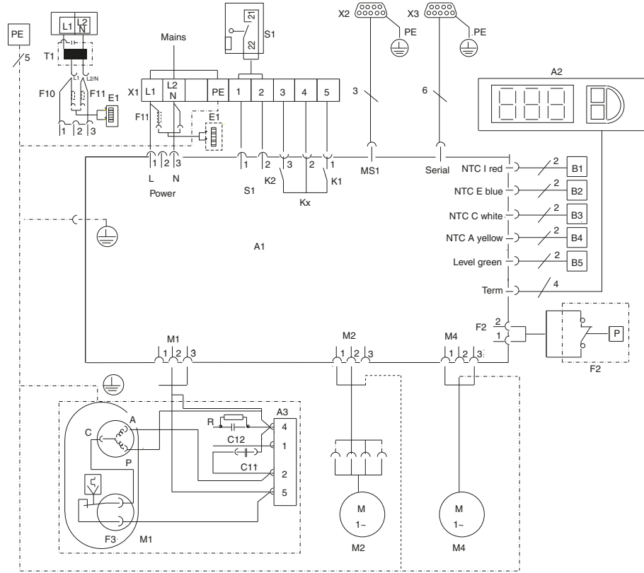
Fig. 27: Esquema de conexões elétricas nº 5
