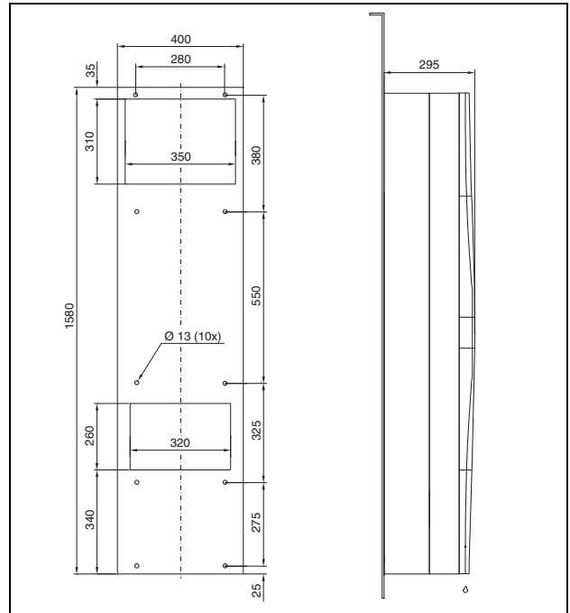
Fig. 129: 3328.xxx, 3329.xxx para montagem externa (exceto os aparelhos NEMA 4X)
