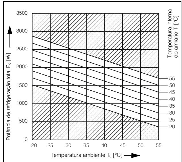
Fig. 100: 3366.xxx (plano), 1500 W, 60 Hz
