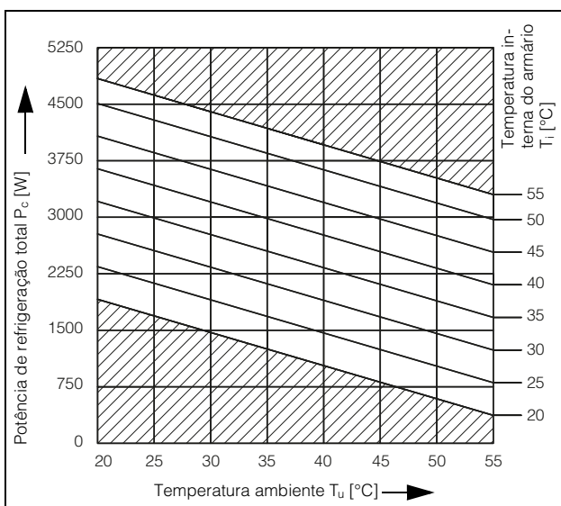
Fig. 103: 3329.xxx, 2500 W, 50 Hz
