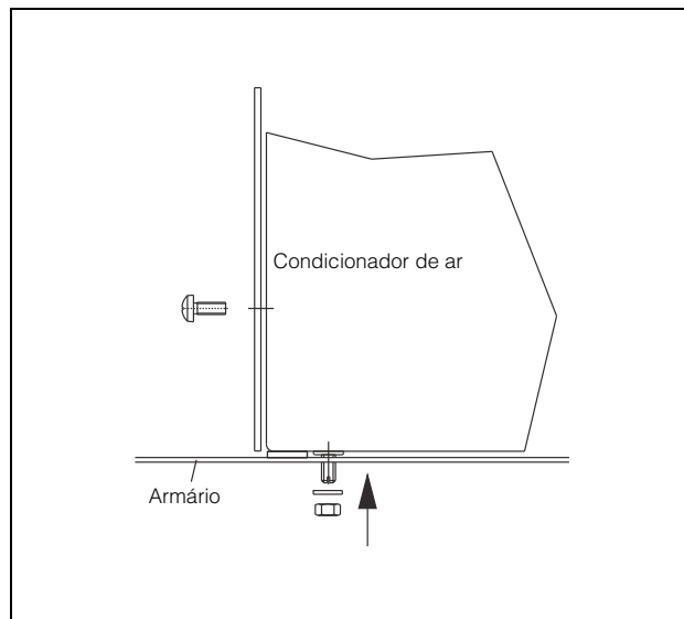
Fig. 83: Montagem do aparelho
