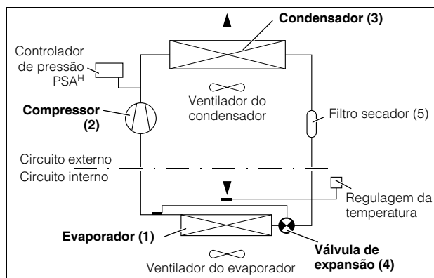
Fig. 3: Circuito de refrigeração
