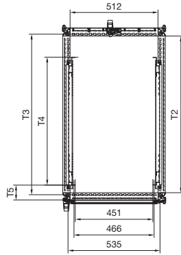
Kesit A – A, genişlik 600 mm
