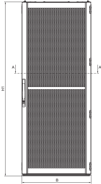
Önden görünüş
