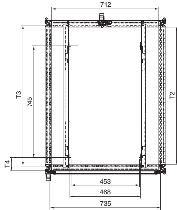
Kesit A – A genişlik 800 mm
