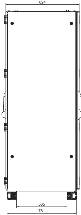
Yandan görünüş
