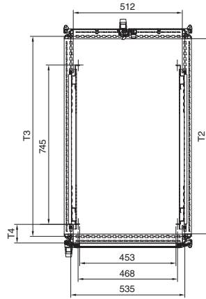
Kesit A – A genişlik 600 mm
