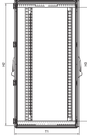
Kesit A – A, genişlik 600 mm
