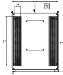
Üstten görünüş
