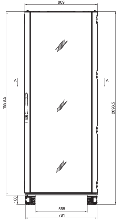
Önden görünüş
