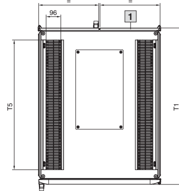
Üstten görünüş
