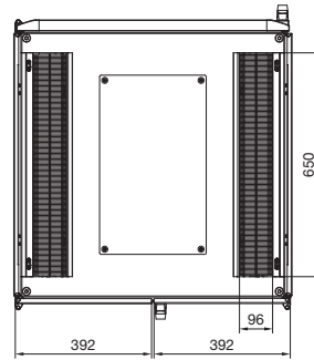
Üstten görünüş
