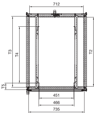
Разрез А – А, IP 55
