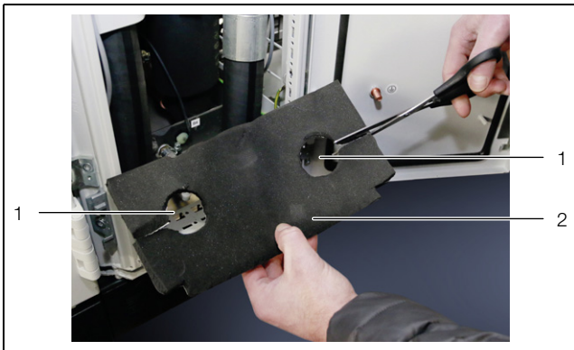
Fig. 2 : Préparation du matériau d'étanchéité
