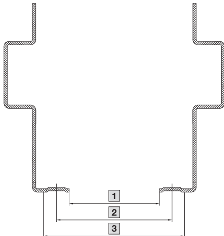
Profil TS IT vzadu
