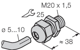
Kabelverschraubung M20 x 1,5
