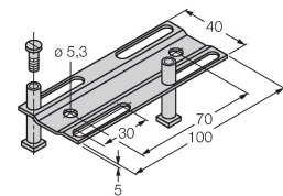
Justierschiene für Quaderbauform CK40 / CP40; Werkstoff: VA 1.4301
