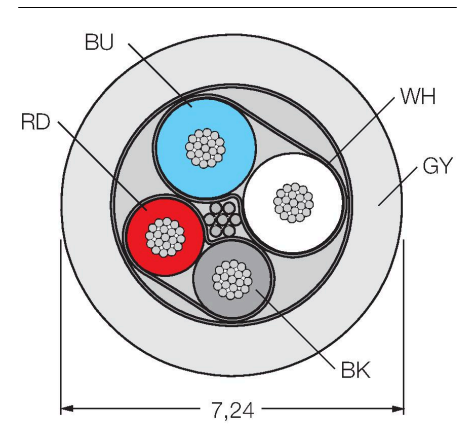
Anschlussbelegung links
