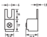
Maßzeichnung Einspeiseklemmen AS 25-Gi
