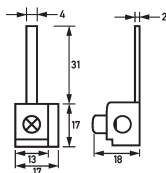
Maßzeichnung Einspeiseklemmen AS 25-SLi
