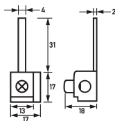
Maßzeichnung Gruppenansicht
