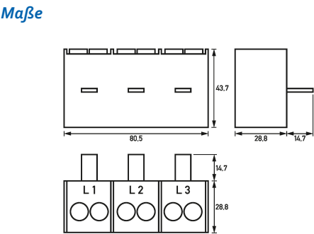
Maßzeichnung Einspeiseklemmen DK Do
