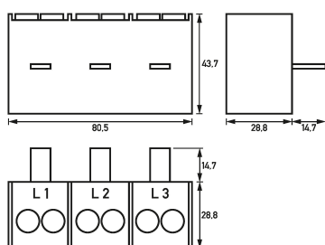
Maßzeichnung Gruppenansicht
