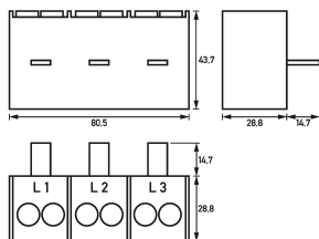
Maßzeichnung Gruppenansicht
