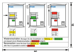
Maßzeichnung Gruppenansicht
