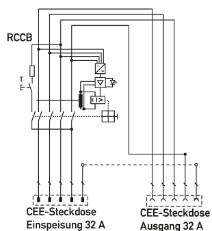
Schaltungsbeispiel Verteiler DPB 32 01-010
