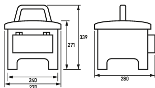
Maßzeichnung Verteiler DPB 32 01-010
