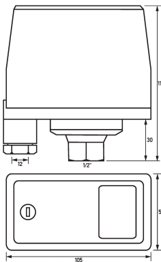
Maßzeichnung Gruppenansicht
