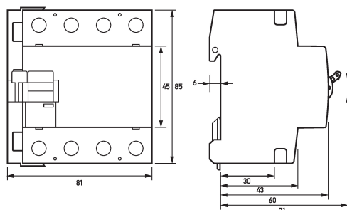
Maßzeichnung Lasttrennschalter DHS 4-063 NA
