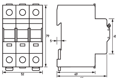
Maßzeichnung Gruppenansicht
