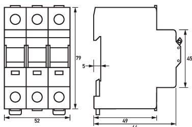
Maßzeichnung Lasttrennschalter RH 025-300
