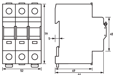
Maßzeichnung Lasttrennschalter RH 063-300
