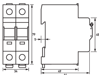
Maßzeichnung Lasttrennschalter RH 100-200
