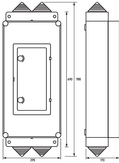
Maßzeichnung Gruppenansicht
