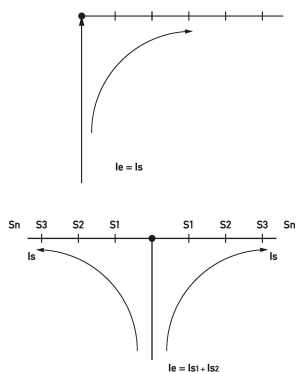
Diagramme Verdrahtungsmaterial B G12TE-1/N/S-10
