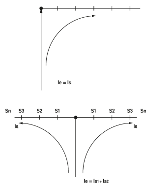
Diagramme Verdrahtungsmaterial EV-S G 2.12.120
